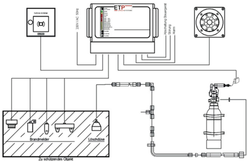
Anlagenschema
